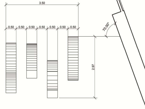
SECCIÓ e:1/50
