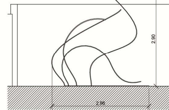
SECCIÓ e:1/50
